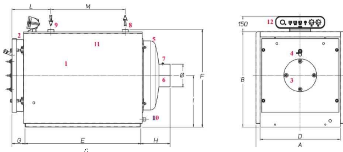
Рисунок 2.2 Схема котла КСМ-240 1 - корпус котла, 2 - передняя часть котла с дверцей с двойным открытием, 3 - ответный фланец для крепления горелки, 4 - окошечко для наблюдения за пламенем, 5 - задняя камера уходящих газов, 6 - дымоход, 7 - отверстие для измерения температуры газов, 8 - присоединение подачи воды в установку, 9 - присоединение возврата воды из установки, 10 - дренаж, 11 - углубление для приборов, 12 - приборная панель
