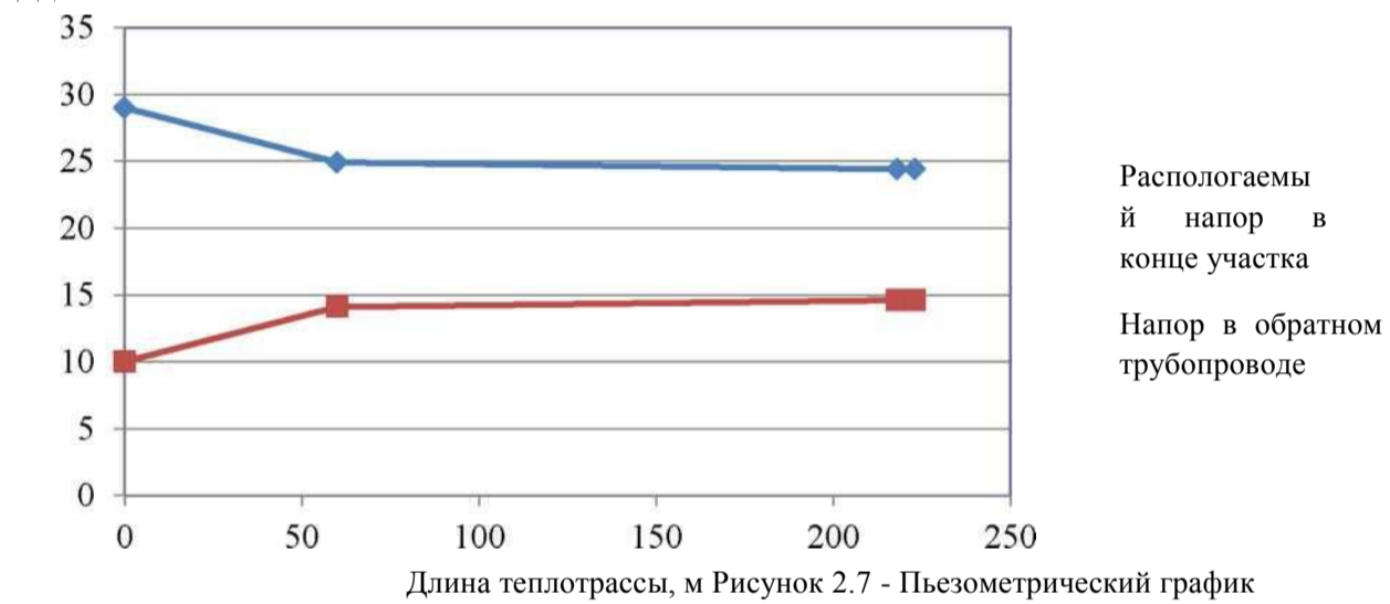
Рисунок 2.6 - Пьезометрический график тепловой сети Котельной с. Петровское по первому магистральному выводу: котельная - больница
