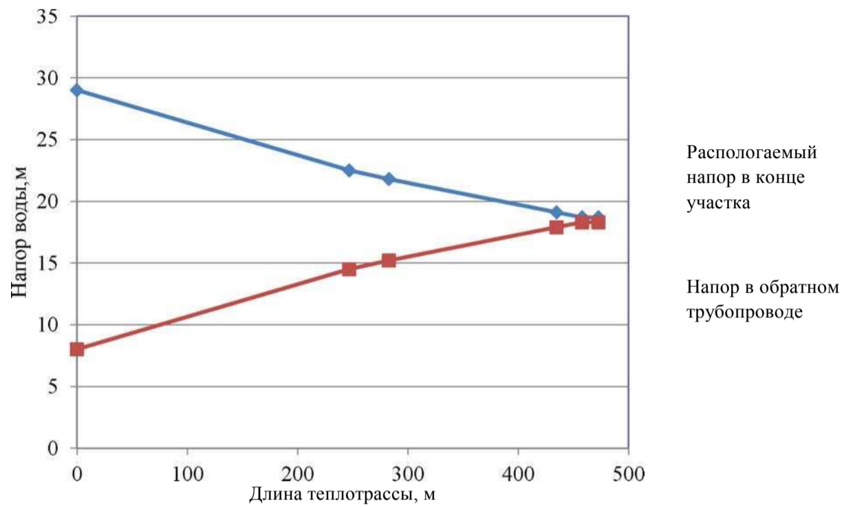
Рисунок 2.13 - Пьезометрический график тепловой сети Котельной с. Малое Шумаково
