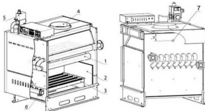
Рисунок 2.4 Устройство котла К.8-А 1 - оребренная труба теплообменника, 2 - теплоизоляция, 3 - рожок горелки, 4 - выход дымовых газов, 5 - газовый клапан, 6 - датчик тяги, 7 - отверстие для замера параметров отходящего газа
