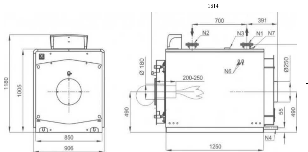
Рисунок 2.1 Схема котла КЕХ-30 N1 - присоединение прямого потока БК 65, N2 - присоединение обратного потока БК 65, N3 - штуцер для приборов 1", N4 - соединение дренажа 1", N5 - присоединение предохранительных клапанов (отсутствуют), N6 - гильзы под термостаты ^ (находится под обшивкой котла), N7 - присоединение термометра ^
