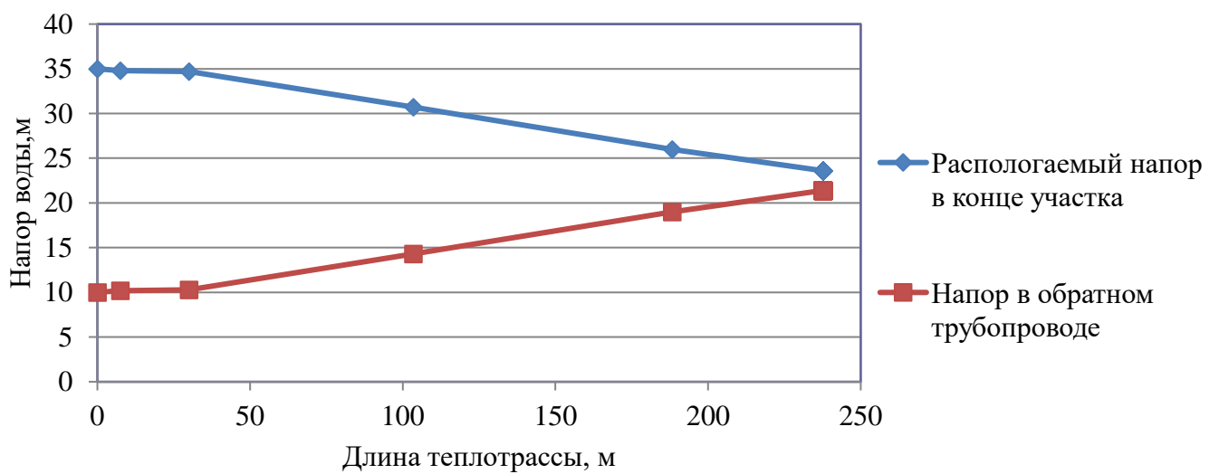
Рисунок 2.8 – Пьезометрический график тепловой сети БМК п. Березовка А-до административного здания, Б-до жилого дома №16
