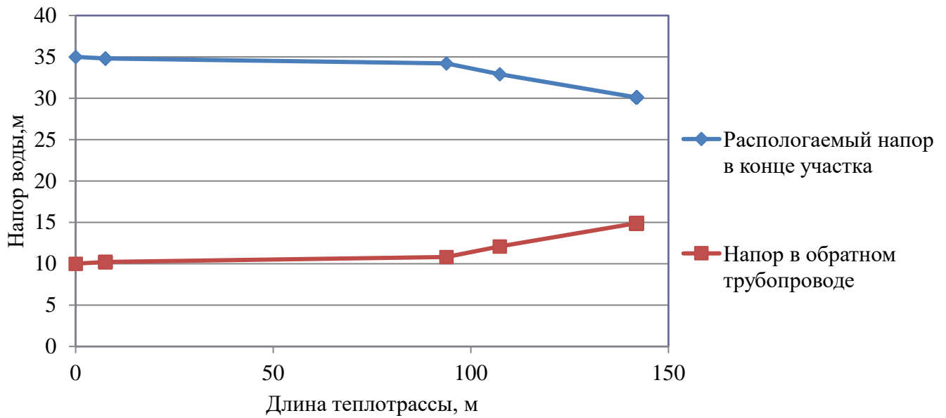
Рисунок 2.11 – Пьезометрический график тепловой сети БМК п. Березовка до здания школы
