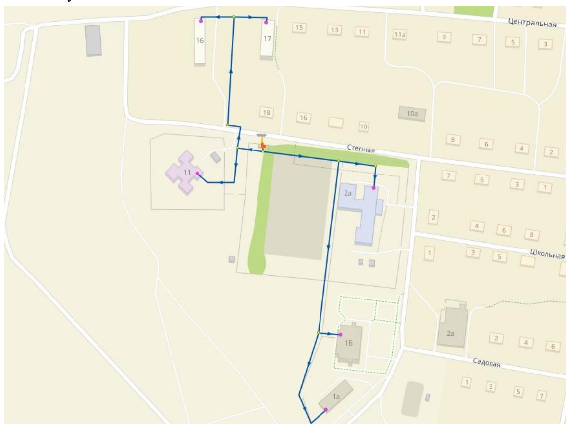
Рисунок 2.15 – Модель системы теплоснабжения БМК п. Березовка
