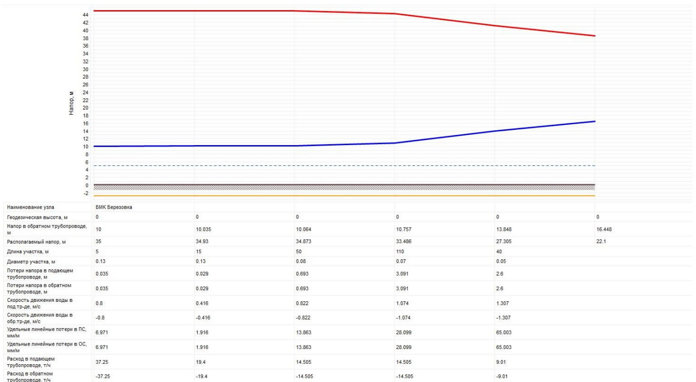
Рисунок 2.19 – Пьезометрический график от источника теплоснабжения (БМК п. Березовка) до жилого дома №16 в аварийной ситуации
