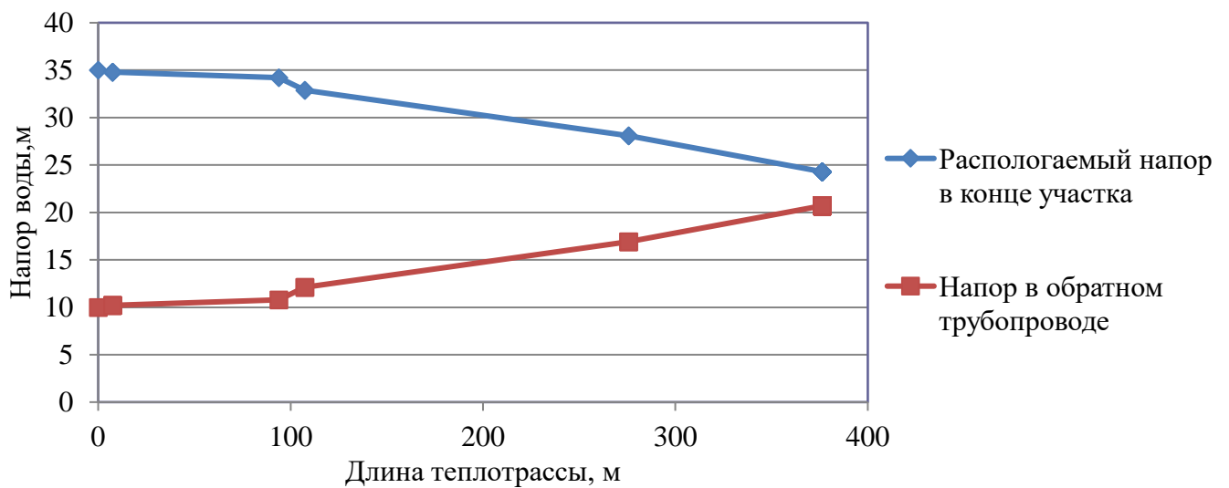
Рисунок 2.7 – Пьезометрический график тепловой сети Котельной п. Каменский
