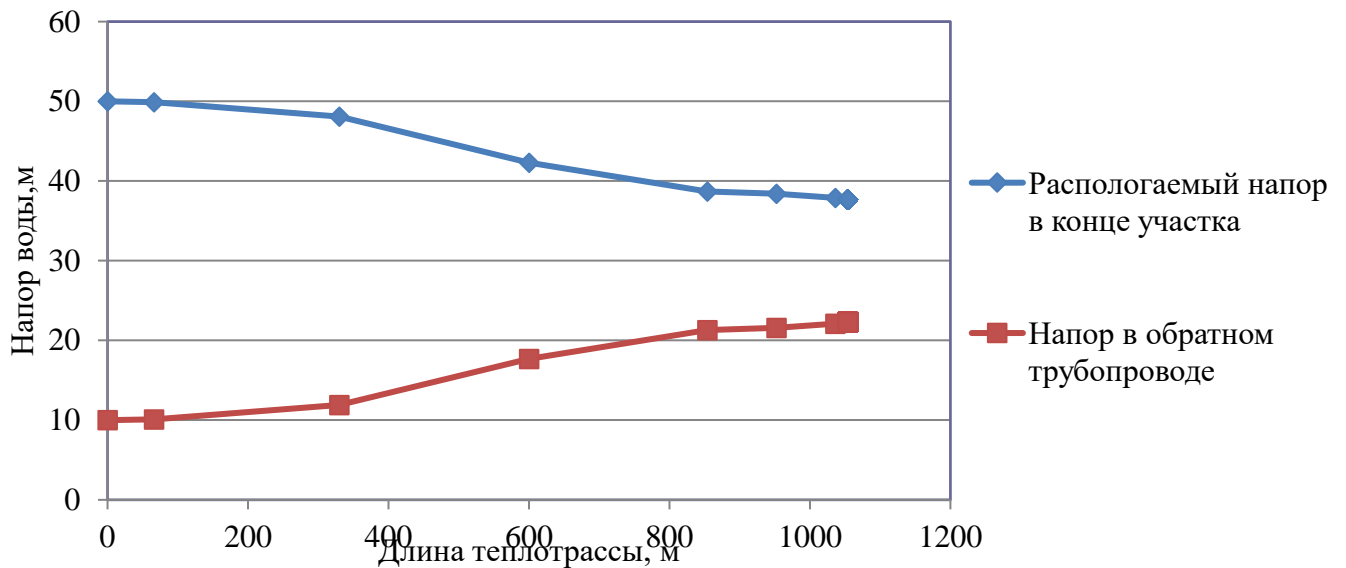
Рисунок 2.7 – Пьезометрический график тепловой сети Котельной п. Каменский
