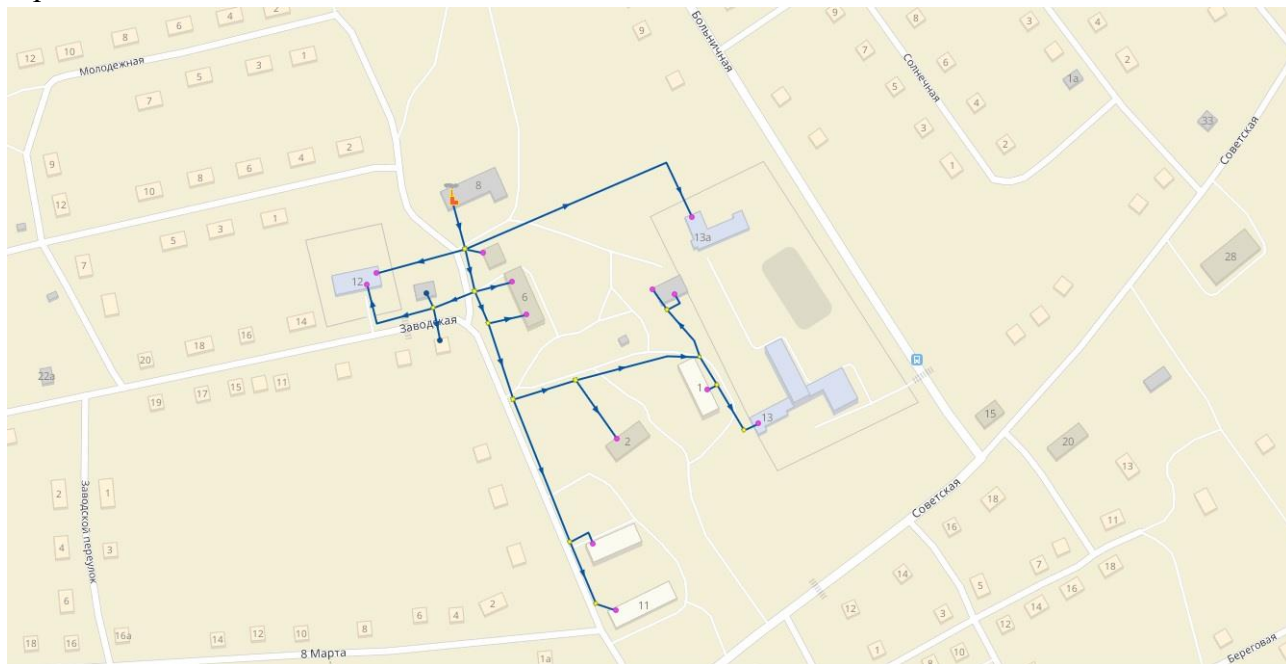
Рисунок 2.14 – Модель системы теплоснабжения Котельной п. Каменский
