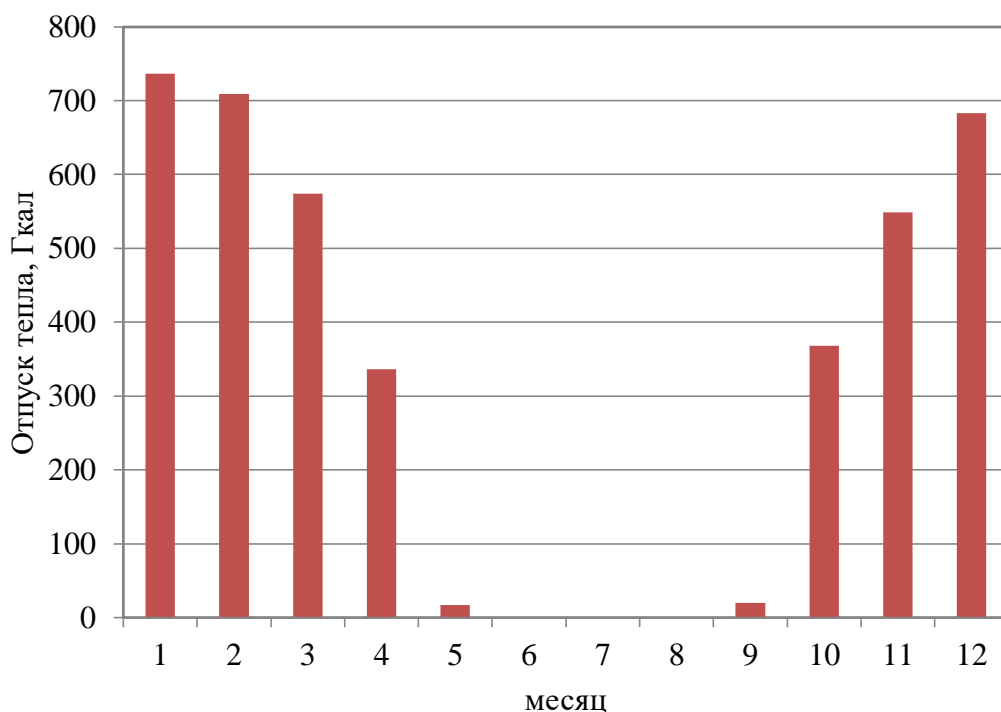
Рисунок 1.5 – Оптимальный температурный график отпуска тепловой энергии на отопление для котельной с. Хомутинино
