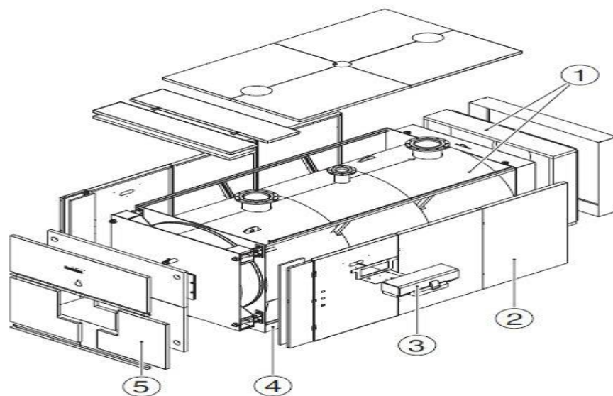
Рисунок 2.1 – Схема котла buderus logano sk745-1200
