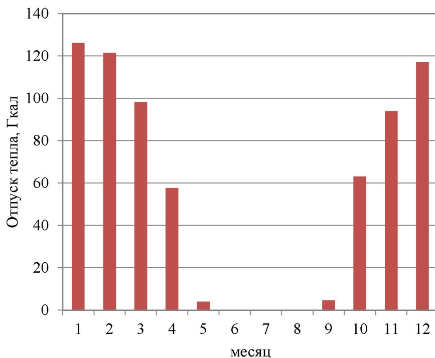
Рисунок 1.4 – Оптимальный температурный график отпуса тепловой энергии для котельной с. Половинка с температурным режимом 95-70 °С
