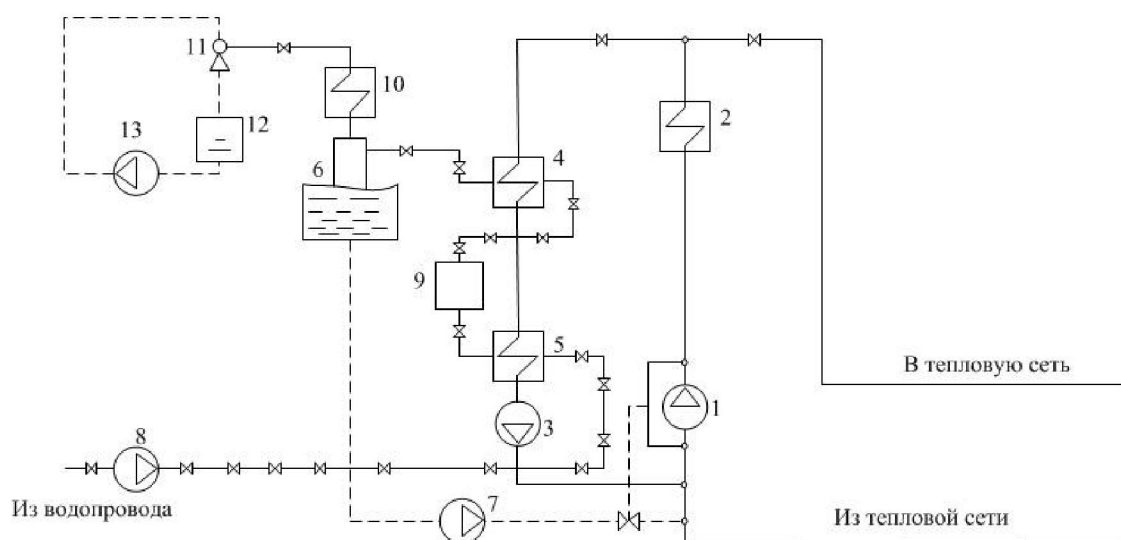
Рисунок 2.5 – Принципиальная тепловая схема котельной с водогрейными котлами:
