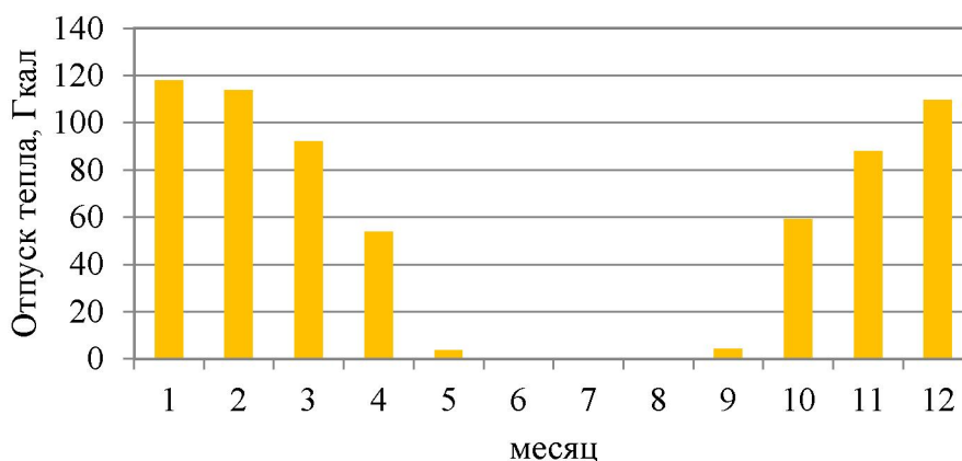
Рисунок 1.5 – Оптимальный температурный график отпуса тепловой энергии для Блочной-котельной д. Водопойка
