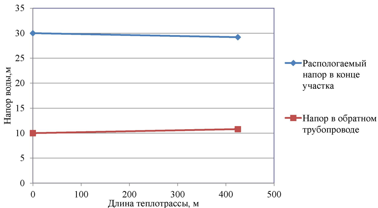
Рисунок 2.9 – Пьезометрический график тепловой сети Блочной-котельной д. Водопойка
