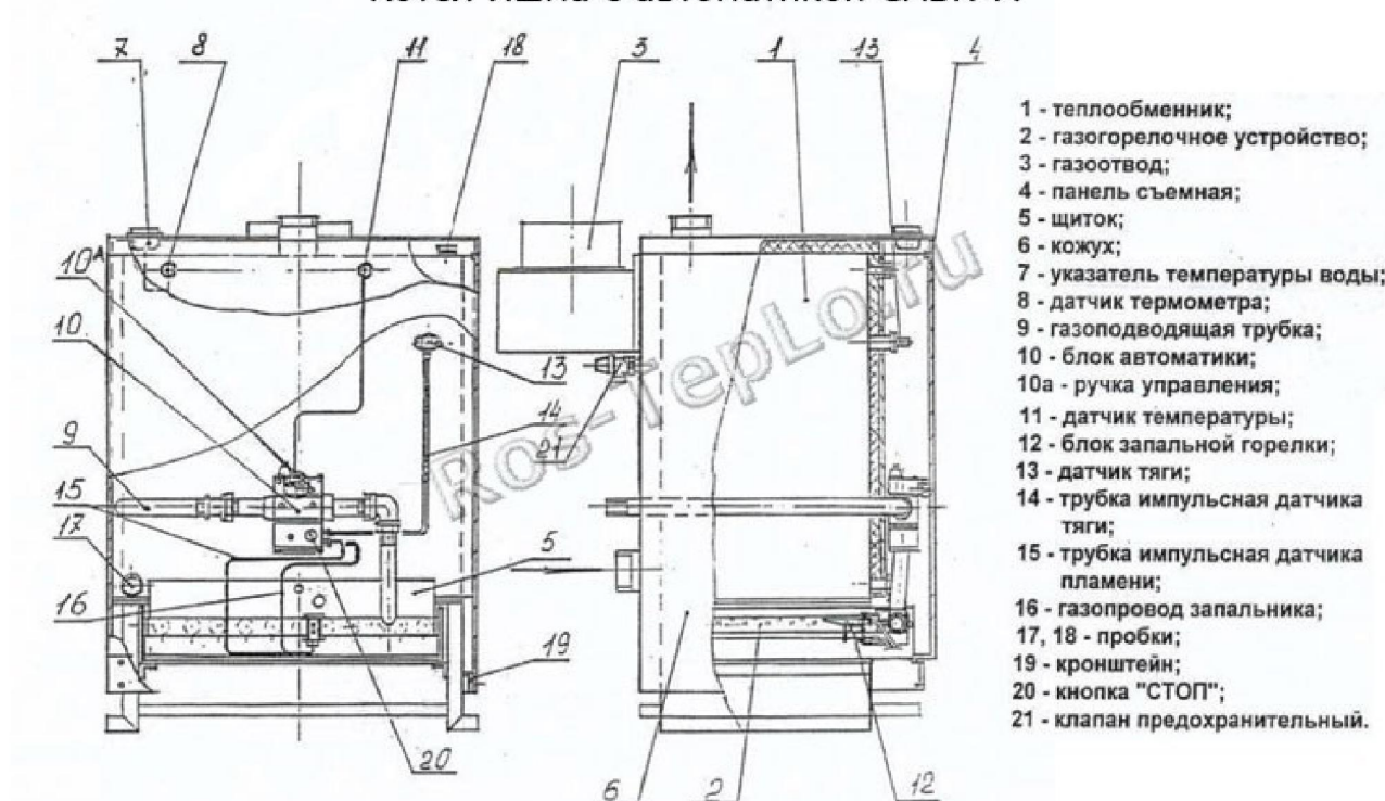
Котел Ишма с автоматикой САБК-М
