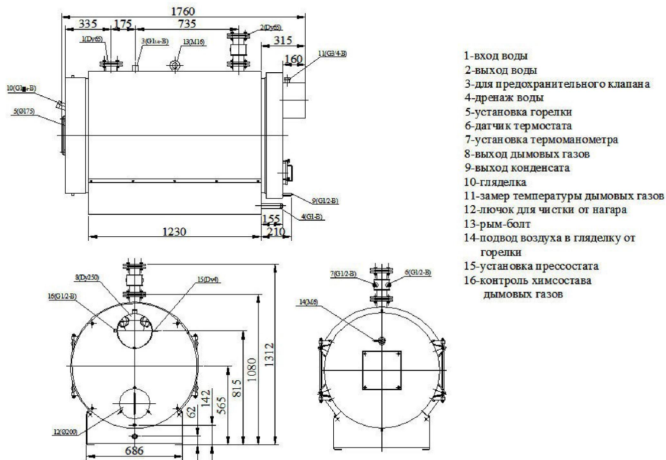
Котел ЗиОСаб-250 ГОСТ 30735-2001 (КВа-0,250-Г/Лж)
