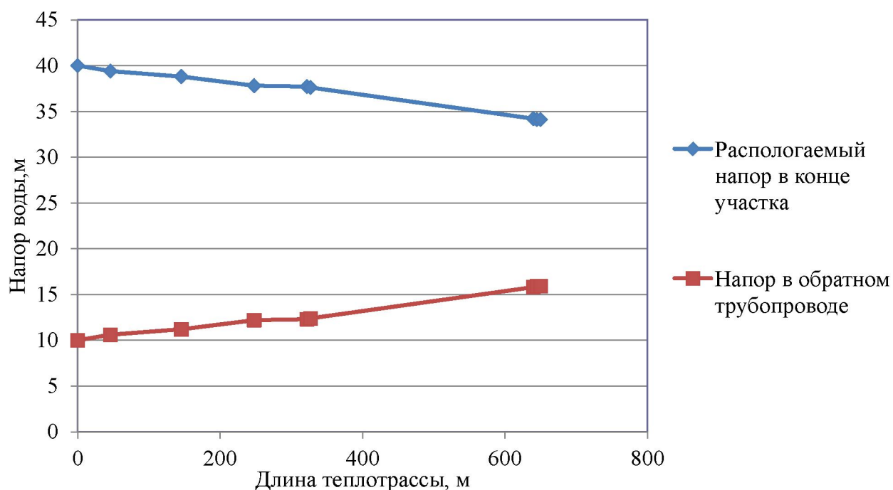
Рисунок 2.7 – Пьезометрический график тепловой сети Котельной с. Половинка
