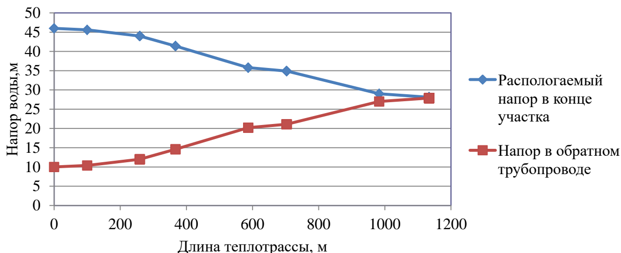
Рисунок 2.19 – Пьезометрический график тепловой сети Котельная п. Нагорный до ул. Молодежная
