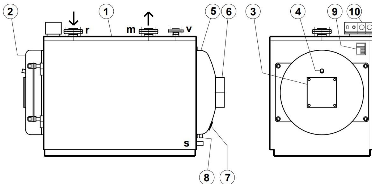
Рисунок 2.1 Устройство котла Super RAG 230
