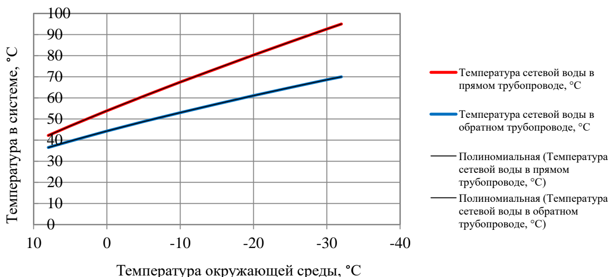
Рисунок 2.6 – График изменения температур теплоносителя 95–70 °C
