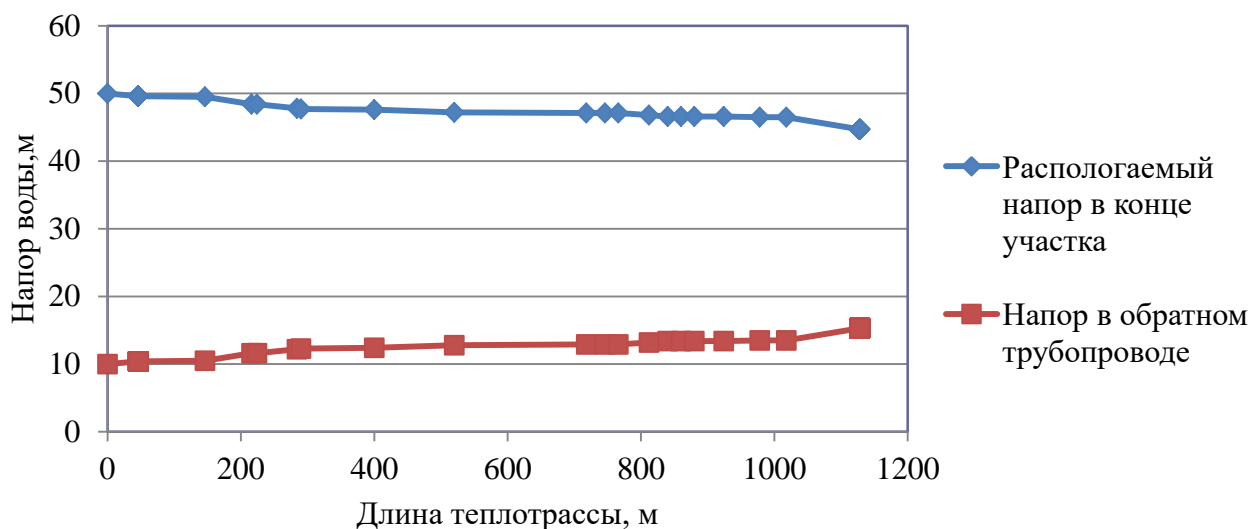
Рисунок 2.9 – Пьезометрический график тепловой сети Котельная №2 с. Кичигино до частных домов по ул. Комсомольская
