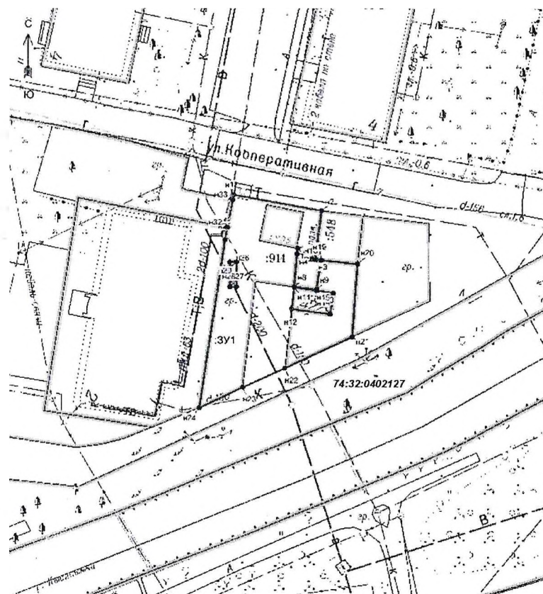
Чертеж межевания территории (:ЗУ1)
