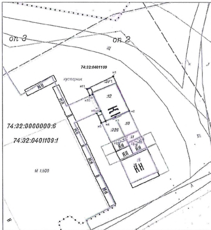
Чертеж межевания территории
