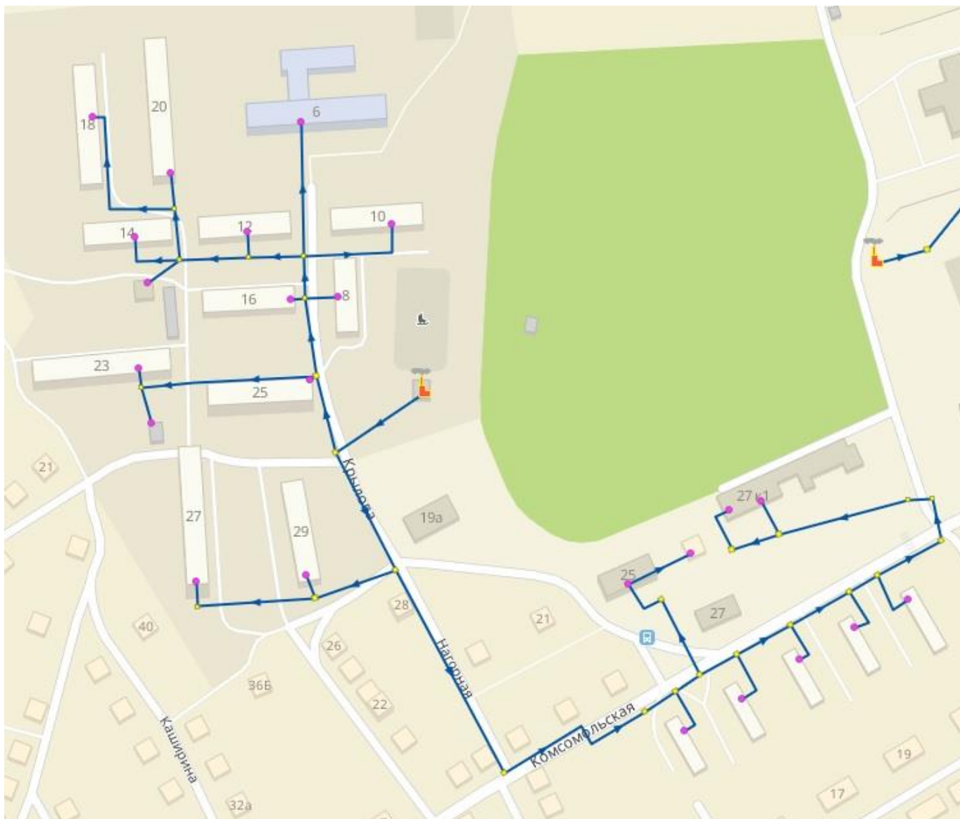
Рисунок 2.29 – Модель системы теплоснабжения Котельной №2 с. Кичигино
