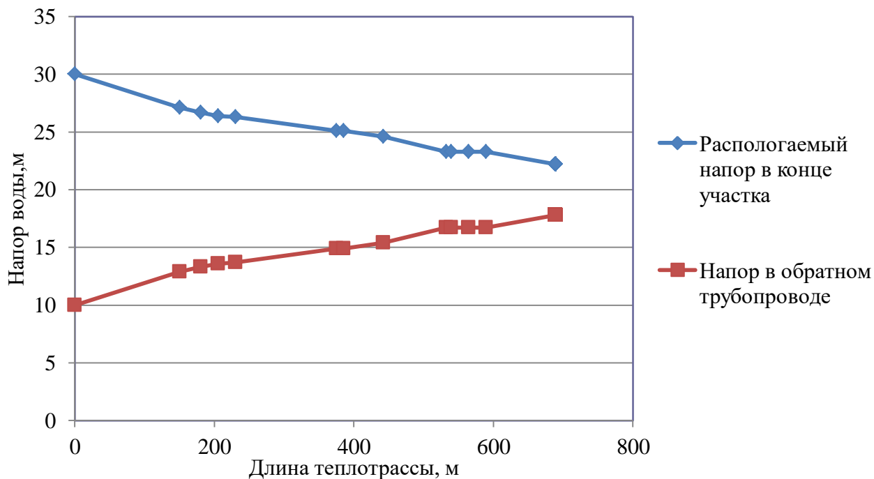
Рисунок 2.14 – Пьезометрический график тепловой сети Котельная п. Синий Бор
