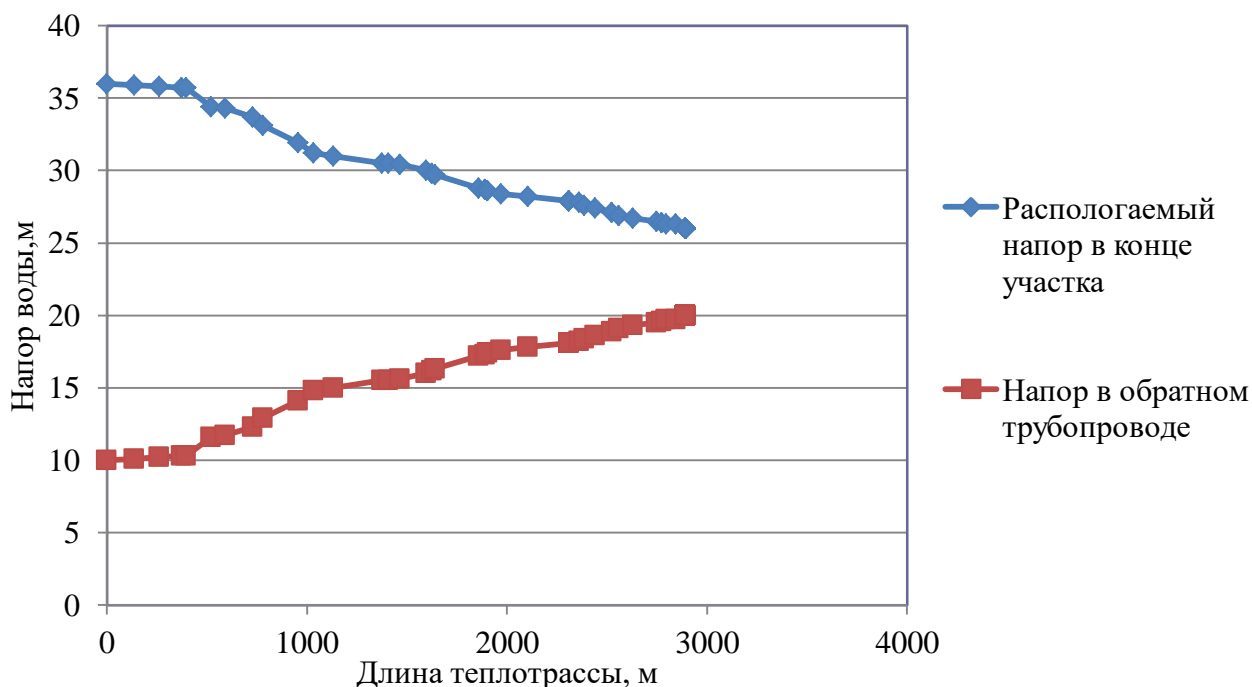
Рисунок 2.9 – Пьезометрический график тепловой сети Котельная п. Нагорный
