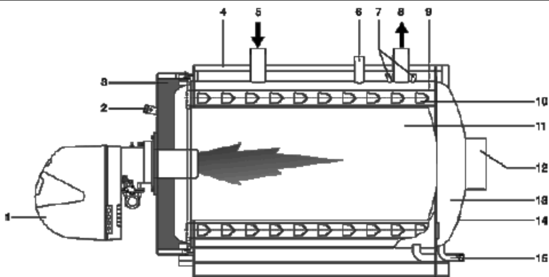
Рисунок 2.1 Устройство котла Riello RTQ
