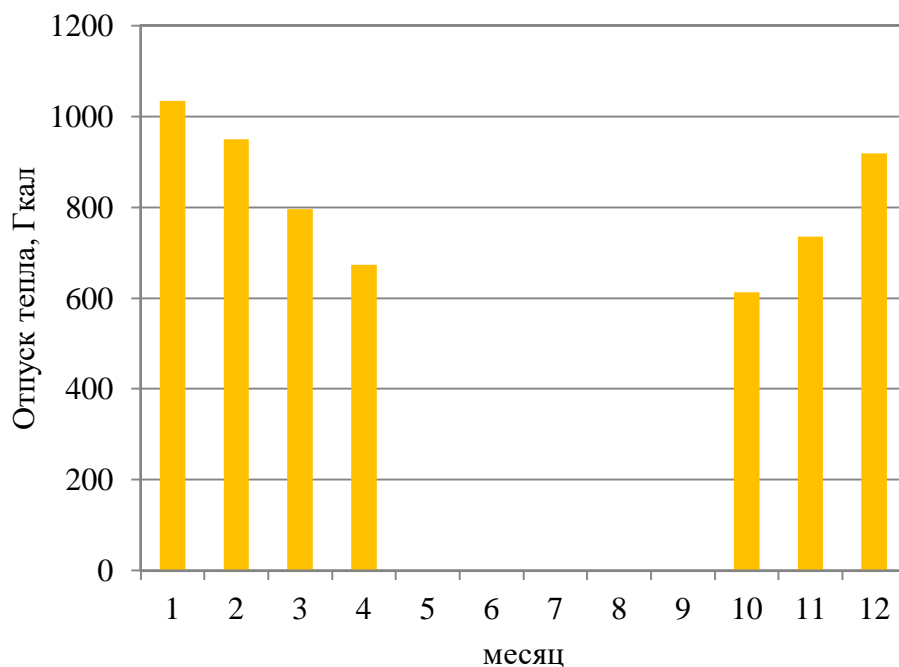
Рисунок 1.6 Оптимальный температурный график отпуса тепловой энергии для Котельная №2 с. Кичигино с температурным режимом 85-64 °С
