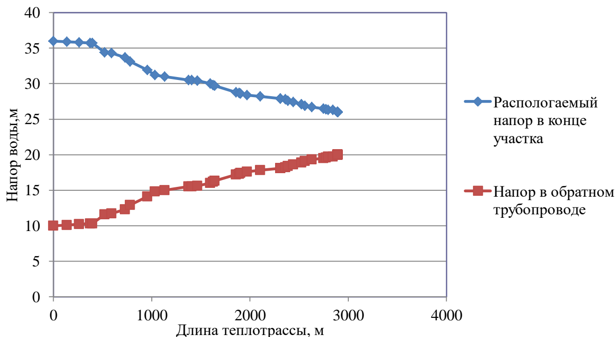
Рисунок 2.13 – Пьезометрический график тепловой сети Котельная п. Нагорный
