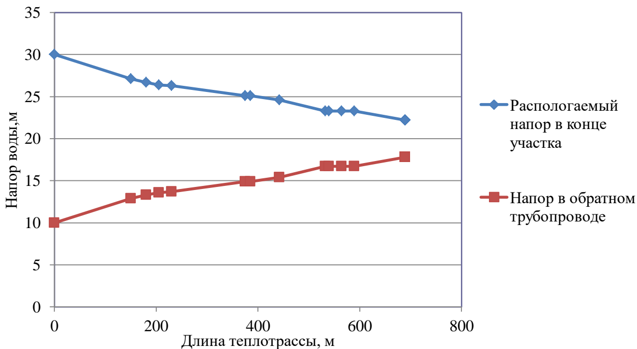
Рисунок 2.10 – Пьезометрический график тепловой сети Котельная п. Синий Бор
