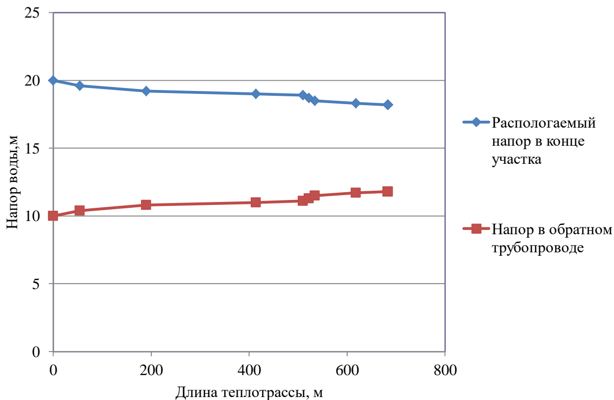
Рисунок 2.11 – Пьезометрический график тепловой сети Котельной №1 с. Кичигино
