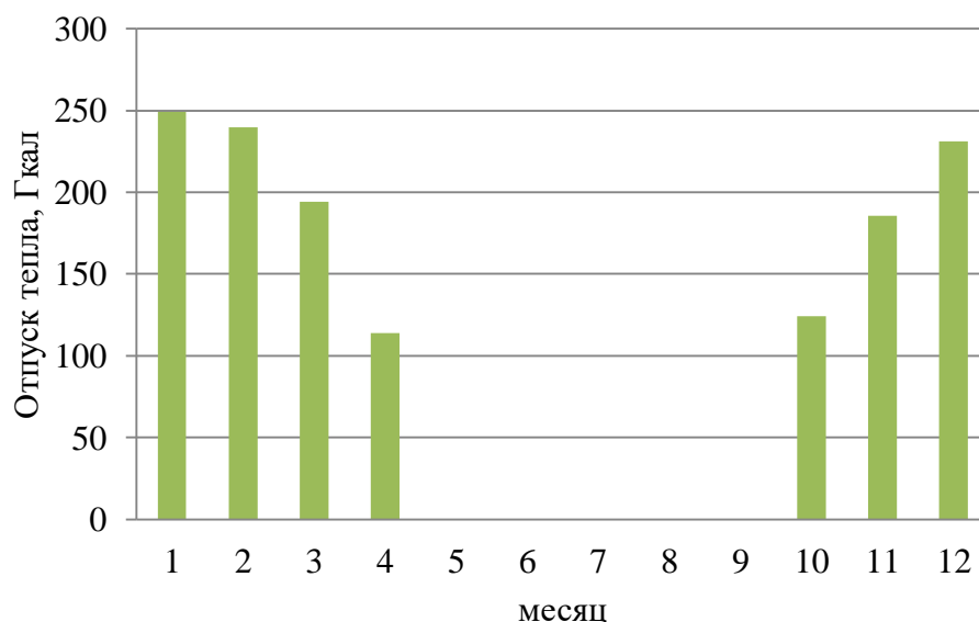
Рисунок 1.8 Оптимальный температурный график отпуски тепловой энергии для Котельная п. Синий Бор с температурным режимом 90-70 °С
