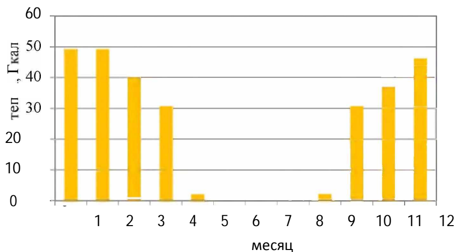
Рисунок 1.5 Оптимальный температурный график отпуска тепловой энергии для Мини-котельная п. Каменский с температурным режимом 85–64 °С
