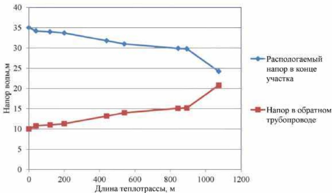
Рисунок 2.10 – Пьезометрический график тепловой сети БМК п. Березовка
