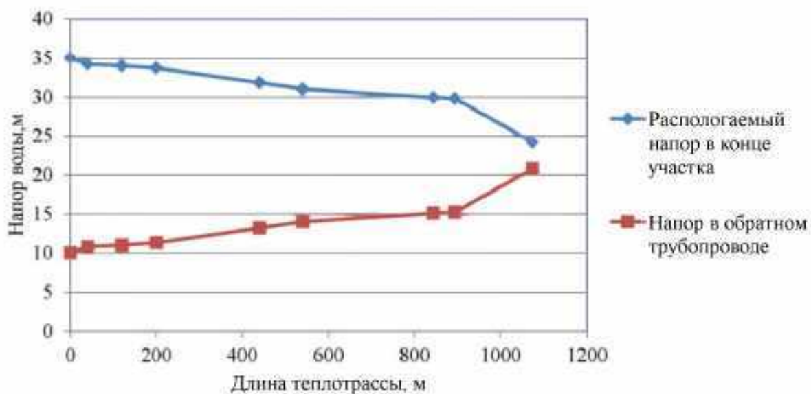
Рисунок 2.8 – Пьезометрический график тепловой сети БМК п. Березовка
