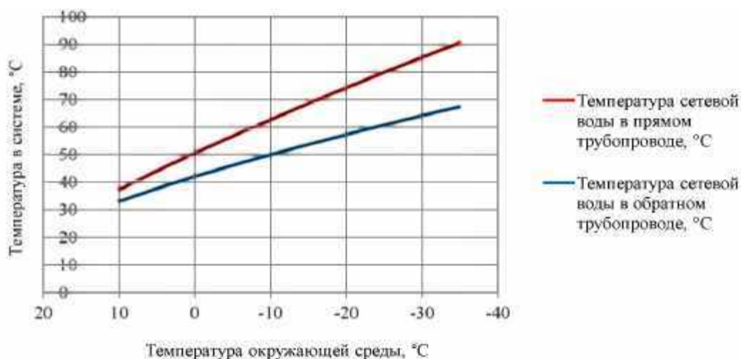
Рисунок 2.5 – График изменения температур теплоносителя 90–70 °С
