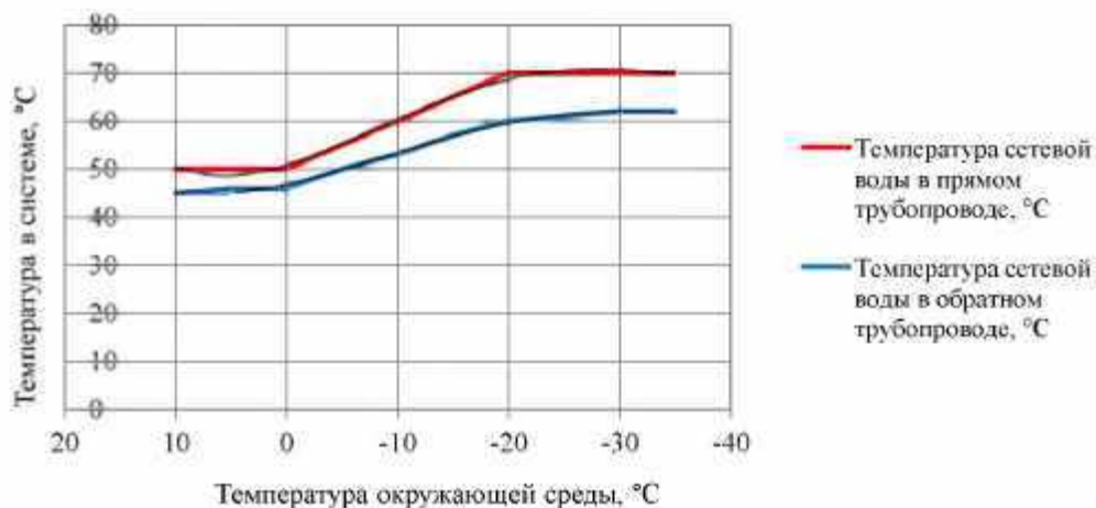
Рисунок 2.6 – График изменения температур теплоносителя 85–64 °С
