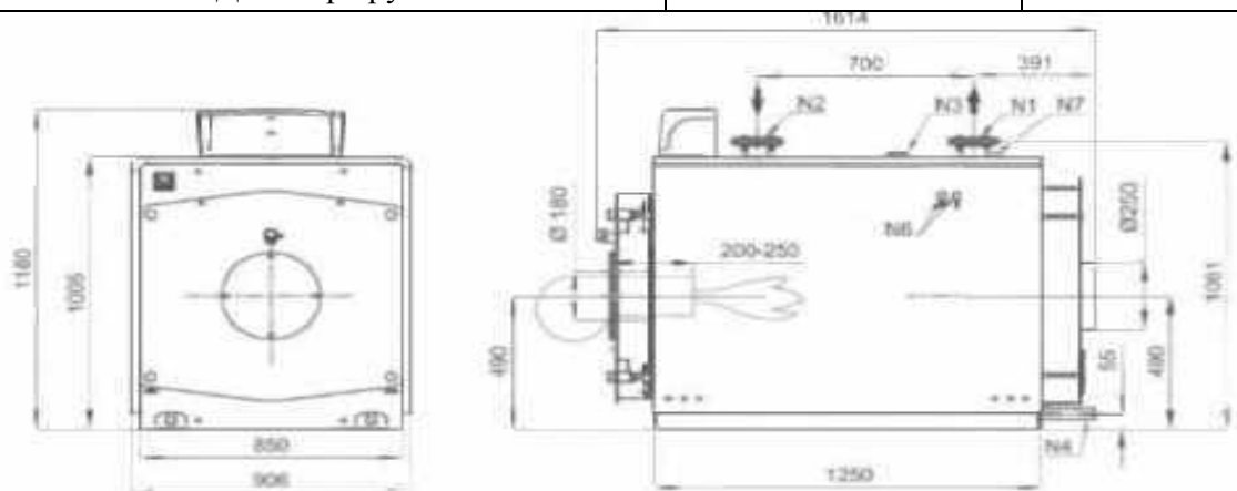
Рисунок 2.3 Общий вид котла ICI REX 62
