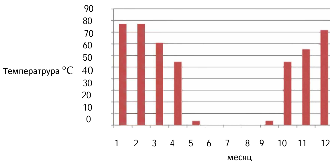
Рисунок 1.4 — Оптимальный температурный график отпуска тепловой энергии для Котельной п. Каменский с температурным режимом 85–64 °С
