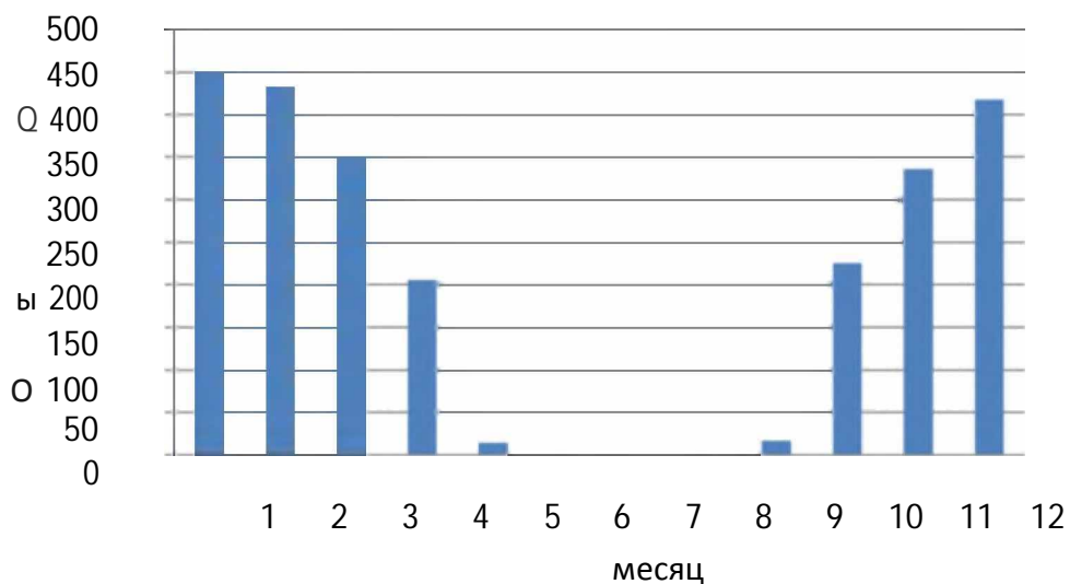
Рисунок 1.6 Оптимальный температурный график отпуска тепловой энергии для БМК п. Березовка с температурным режимом 90–70 °С
