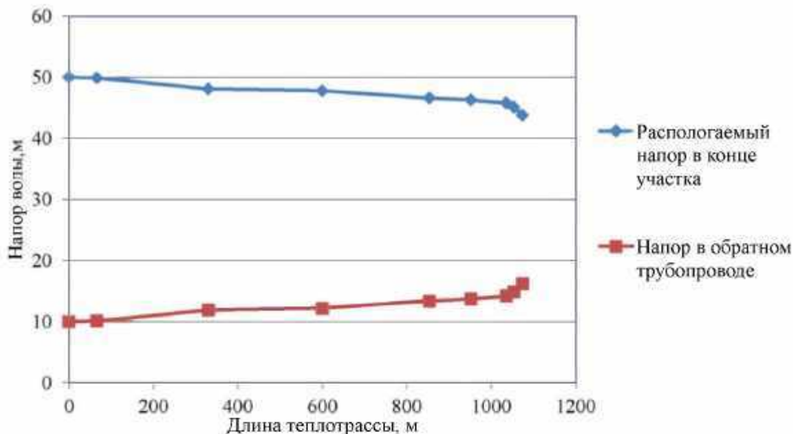
Рисунок 2.9 – Пьезометрический график тепловой сети Котельной п. Каменский
