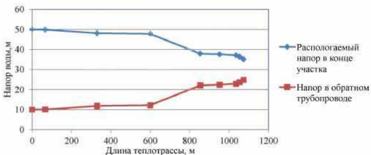
Рисунок 2.7 – Пьезометрический график тепловой сети Котельной п. Каменский
