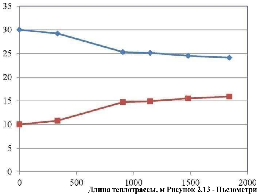
Рисунок 2.13 - Пьезометрический график тепловой сети Котельной с. Хуторка
