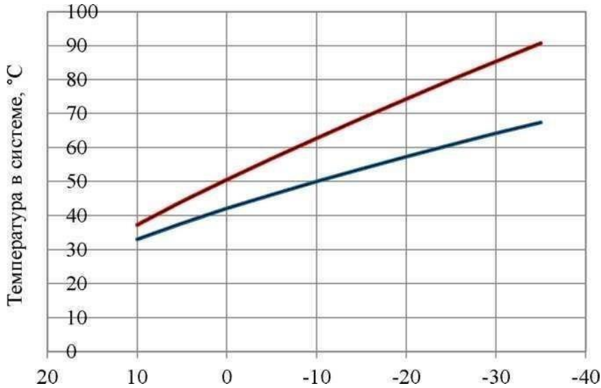
Рисунок 2.7 - График изменения температур теплоносителя 95-70 °С
